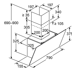
Afmeting in mm Apparaat in luchtafvoermodus
