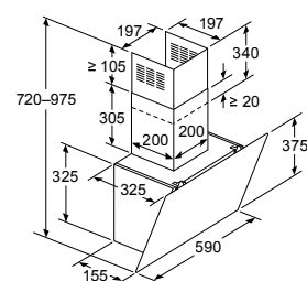
Afmeting in mm Apparaat in luchtcirculatiemodus
