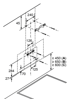
Afmeting in mm Wandinstallatie met luchtkanaal
