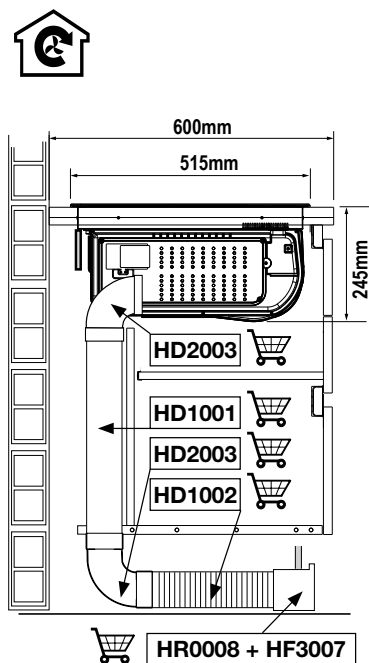
uitvoering 1: Afvoer naar buiten
