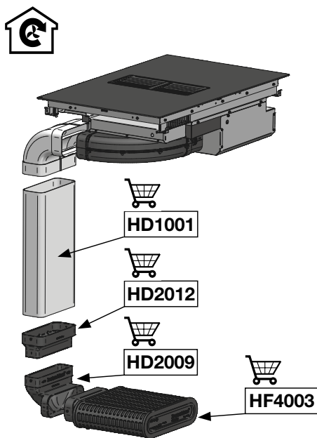
Uitvoering 3, Recirculatie met Plasmafilter onder de kast
