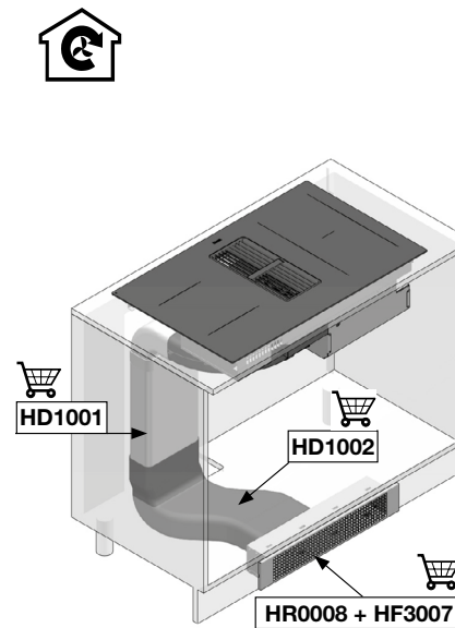
Uitvoering 2, Recirculatie met uitblaas vooraan bij de plint
