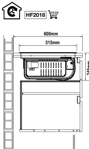
Uitvoering 3: Recirculatie met bodem-achterwand combinatie
