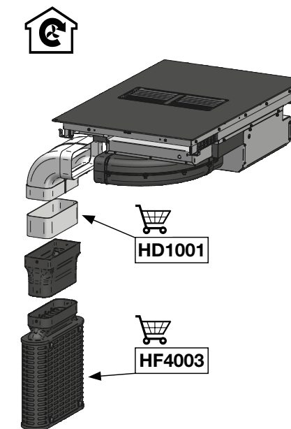
Uitvoering 4, Recirculatie met Plasmafilter achter de kast
