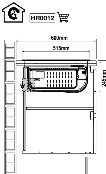
Uitvoering 2: Recirculatie met startset voor uitblaas door de achterwand
