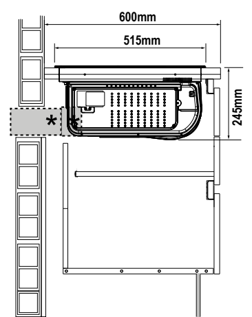
uitvoering 1: Afvoer naar buiten
