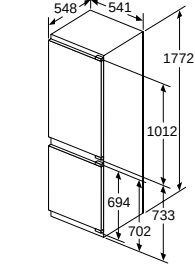
Afmeting in mm
