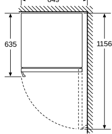
Afmeting in mm
