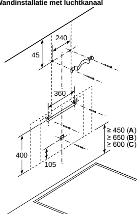
Afmeting in mm Wandinstallatie met luchtkanaal
