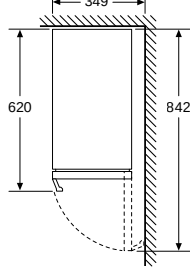
Afmeting in mm
