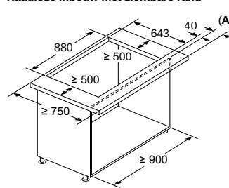
Afmeting in mm Combinatie met elektrische kookplaat Naadloze inbouw met zichtbare rand
