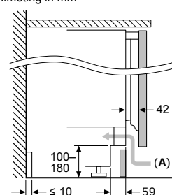
A: Luchtinvoeropening ≥ 200 cm 2
