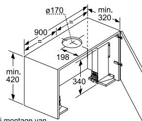
Bij montage van de 90 cm vlakke afzuigkap in een 90 cm brede bovenkast is een montageset noodzakelijk. De beide montagehoeken worden rechts en links in het meubel geschroefd. Montage volgens slabloot. Afmeting in mm
