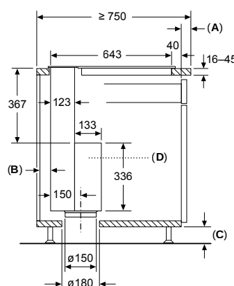
Afmeting in mm Naadloze inbouw met zichtbare rand
