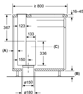
Afmeting in mm Standaard, inbouw met zichtbare rand
