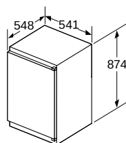
Afmeting in mm
