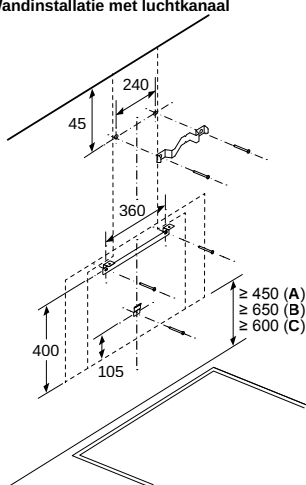
Afmeting in mm Wandinstallatie met luchtkanaal
