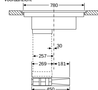
Afmeting in mm Vooraanzicht
