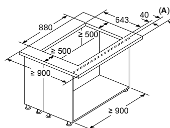
Afmeting in mm Combinatie met elektrische kookplaat Naadloze inbouw met zichtbare rand
