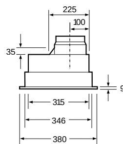
Afmeting in mm
