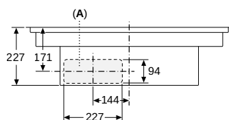
Afmeting in mm Vooraanzicht
