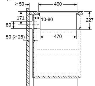
Afmeting in mm Zijaanzicht
