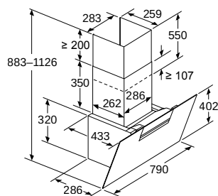
Afmeting in mm Apparaat in luchtafvoermodus
