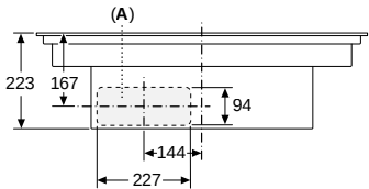
Afmeting in mm Vooraanzicht
