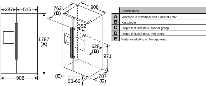
Afmeting in mm
