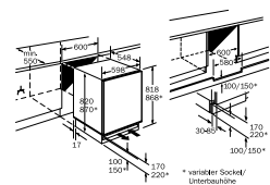
Plaats voor elektrische aansluiting 30cm rechts of links naast het apparaat. Bij een inbouw in de plint.
