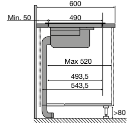
Zijaanzicht werkblad 600 mm
