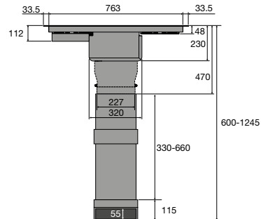
Zijaanzicht werkblad 600 mm combinatie HR0003
