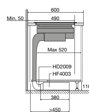
Zijaanzicht met liggend PlasmaMade filter en adapter
