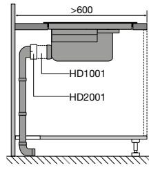
Zijaanzicht verdiept werkblad
