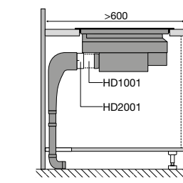
Zijaanzicht verdiept werkblad
