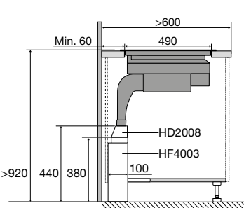
Zijaanzicht met PlasmaMade filter en adapter
