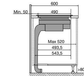
Zijaanzicht werkblad 600 mm
