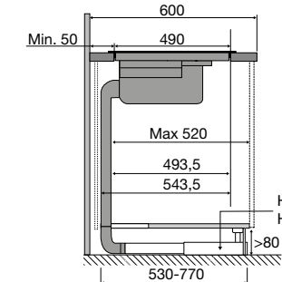
Zijaanzicht werkblad 600 mm combinatie HR0003 en HR0011
