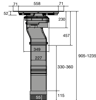
Zijaanzicht werkblad 600 mm combinatie HR0003 en HR0011
