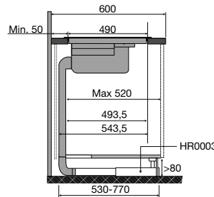
Zijaanzicht werkblad 600 mm combinatie HR0003
